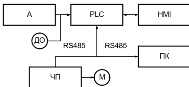
Рис. 6. Схема снятия показаний и регистрации износа зачистного круга Fig. 6. Scheme for taking readings and recording wear on the grinding wheel
