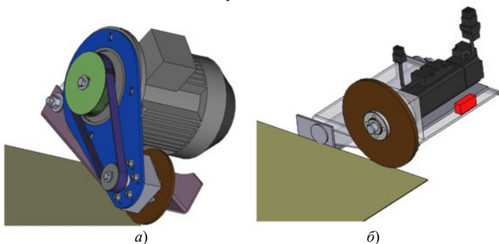
Рис. 2. Конструкции зачистных модулей:
