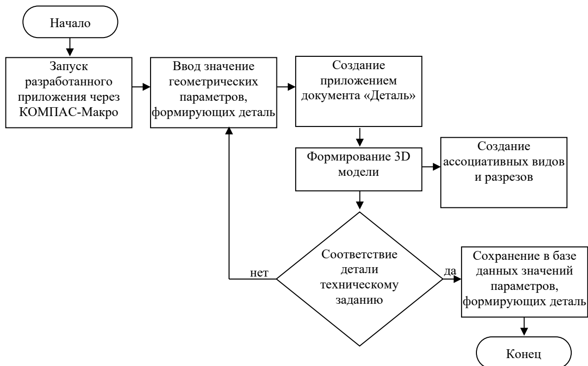
Рис. 5. Блок-схема, поясняющая алгоритм работы с разработанным приложением
