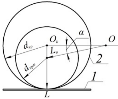
Рис. 4. Схема измерений диаметра круга:
