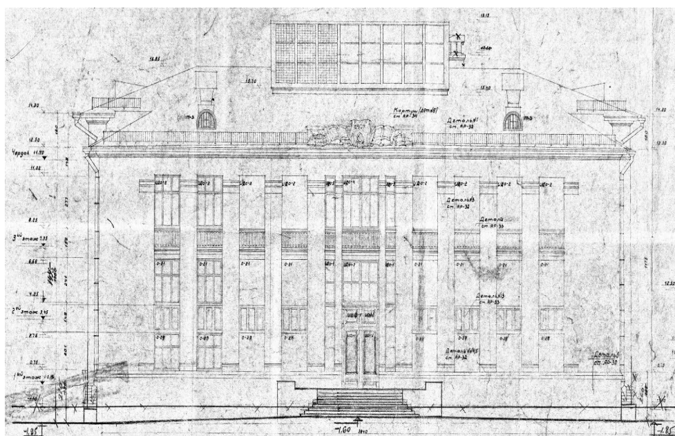
Рис. 10. Проект привязки здания Курской областной библиотеки: главный фасад, архитектор М.Л. Теплицкий (Курскоблпроект), 1956 г.
