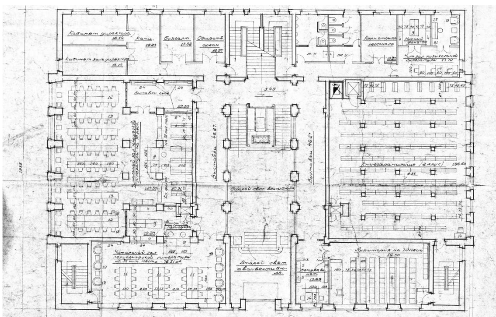
Рис. 7. Проект привязки здания Курской областной библиотеки: первый этаж, архитектор М.Л. Теплицкий (Курскоблпроект), 1956 г.
