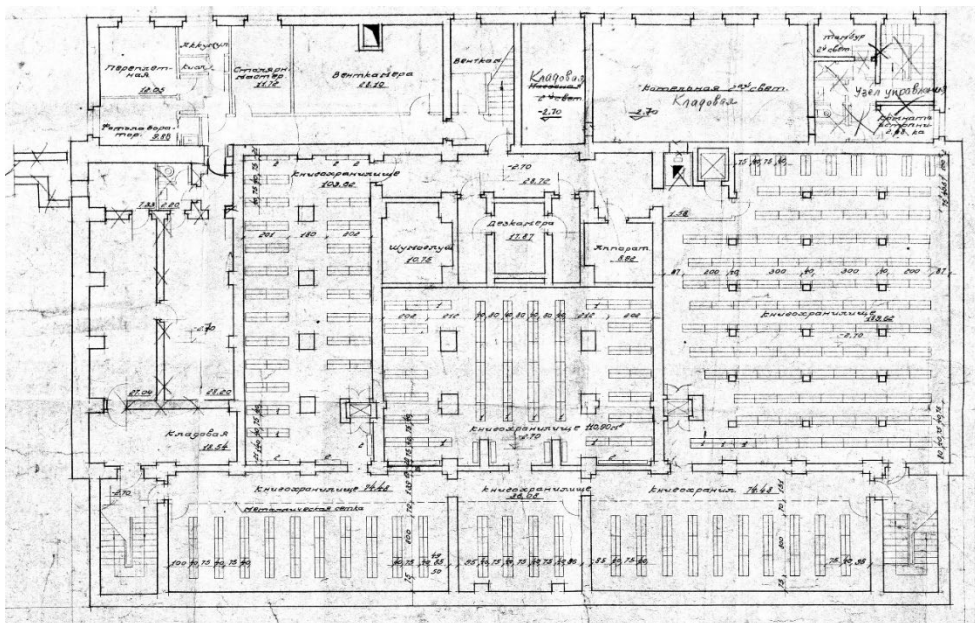
Рис. 6. Проект привязки здания Курской областной библиотеки: подвальное книгохранилище, архитектор М.Л. Теплицкий (Курскоблпроект), 1956 г.
