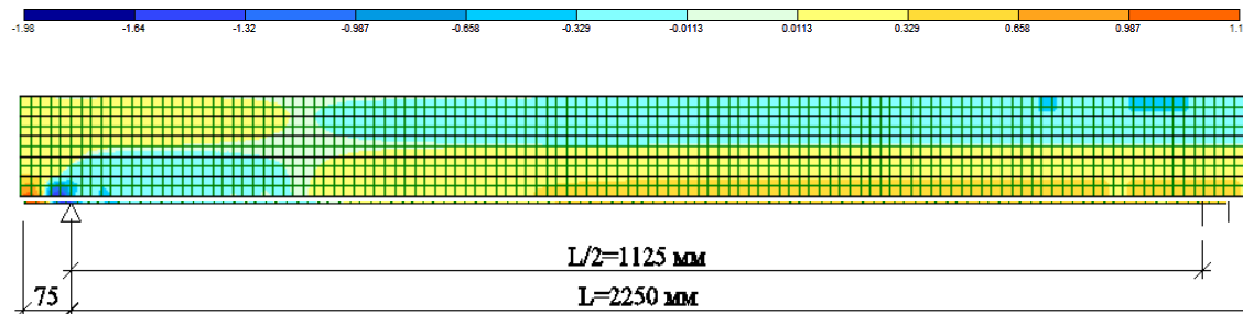
Рис. 3. Эпюра распределения нормальных напряжений при нагрузке 10,4 кН для клеёной балки
