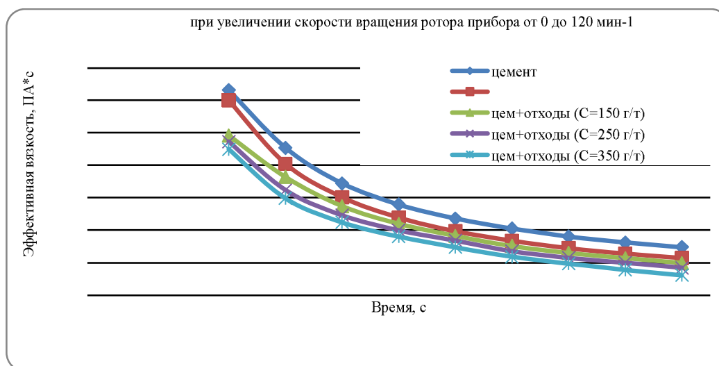
Рис. 1. Изменение эффективной вязкости вязущих композиций различного состава с течением времени при увеличении скорости вращения ротора
