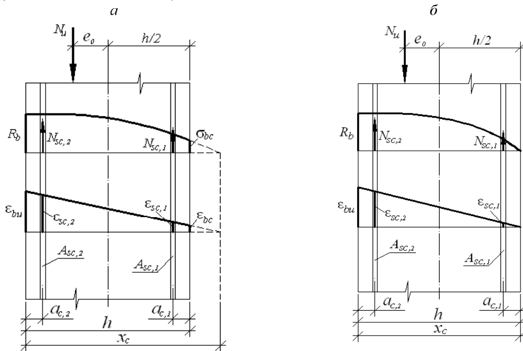
Рис. 1. Схема распределения деформаций, напряжений и усилий в сечении прямоугольного внецентренно сжатого железобетонного элемента на стадии исчерпания его прочности: а – в случае малых эксцентриситетов приложения продольной силы; б – в случае граничного эксцентриситета
